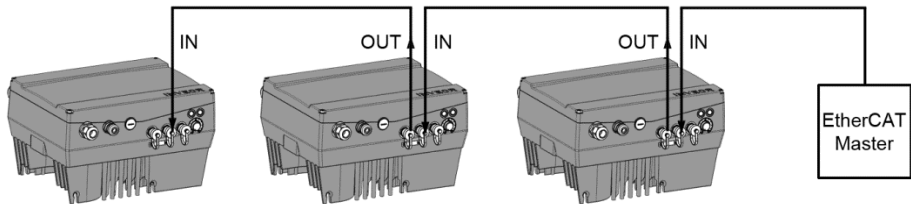
Abb.: 4 Verkabelung und Busanschluss
