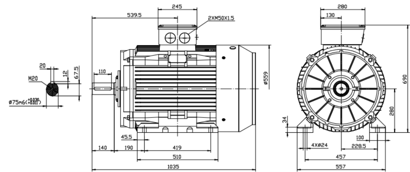
Typ / type IE3 SEV- 280M1-6
